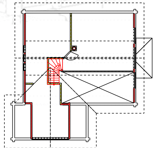
Toinen kerros
