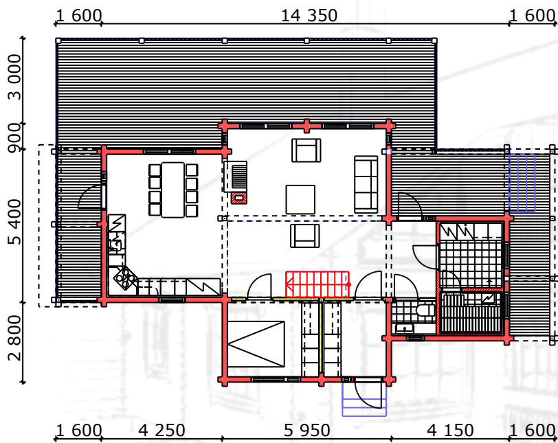
Ensimmäinen kerros
