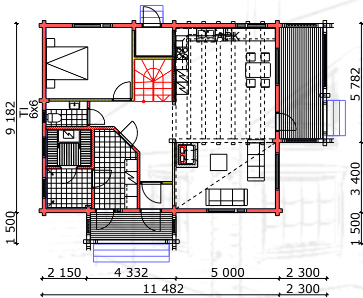
Ensimmäinen kerros
