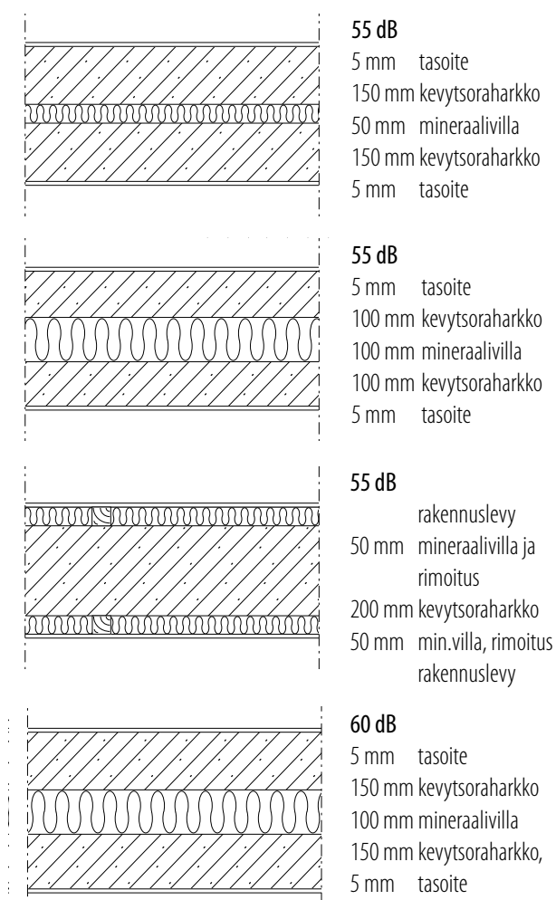
Kuva 2.9. Ilmääneneristysarvoja R'w erilaisilla kevytsoraharkkorakenteilla.
