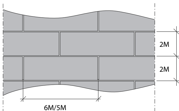
Kuva 3.6. Harkkorakenteiden moduulimitat ovat pystysuunnassa 2M ja pituussuunnassa 6M/5M.
