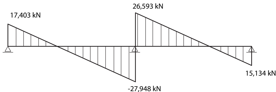
Maanpaineeseinän leikkausvoimapinta
