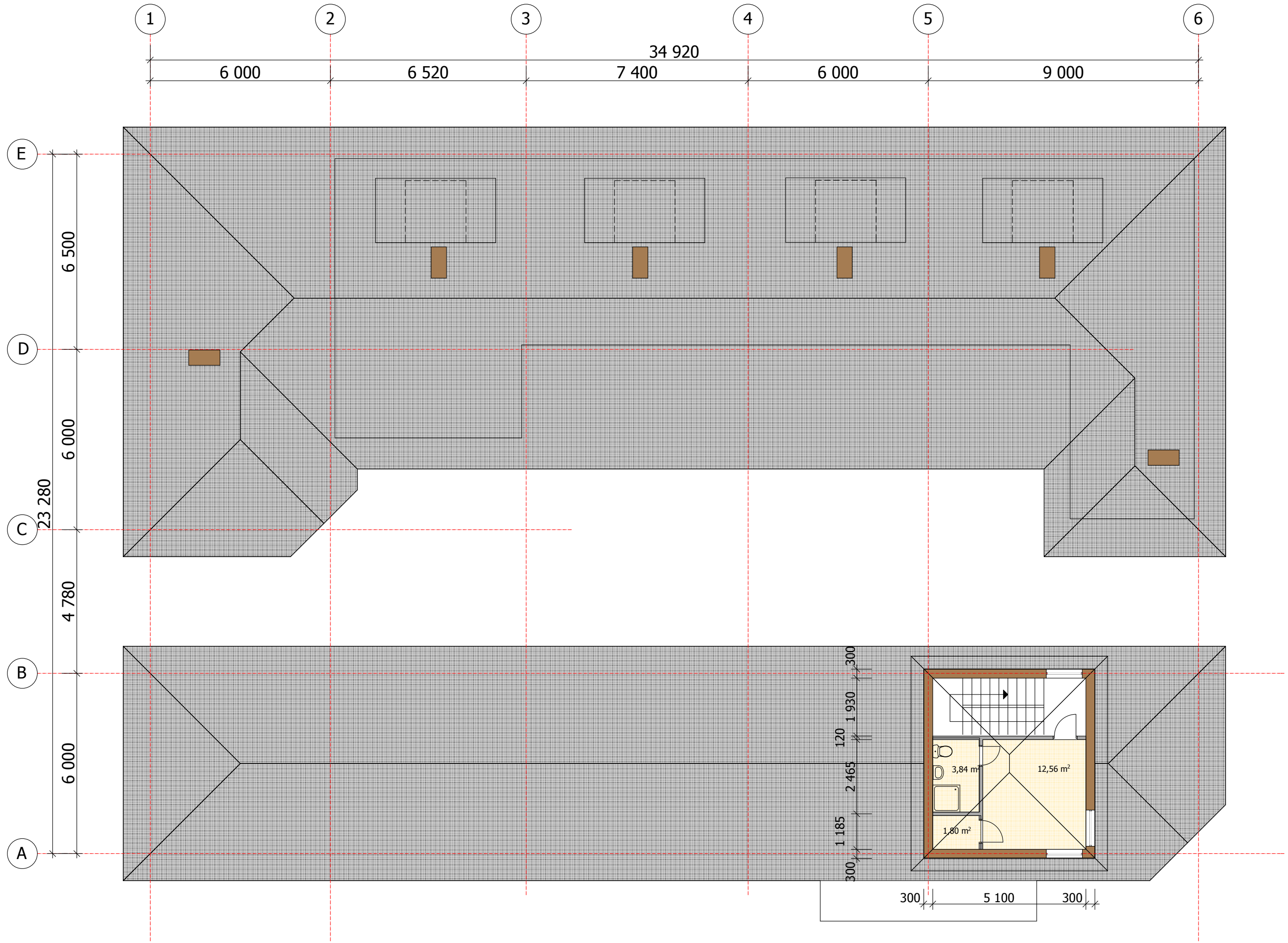
KATUSE PLAAN
